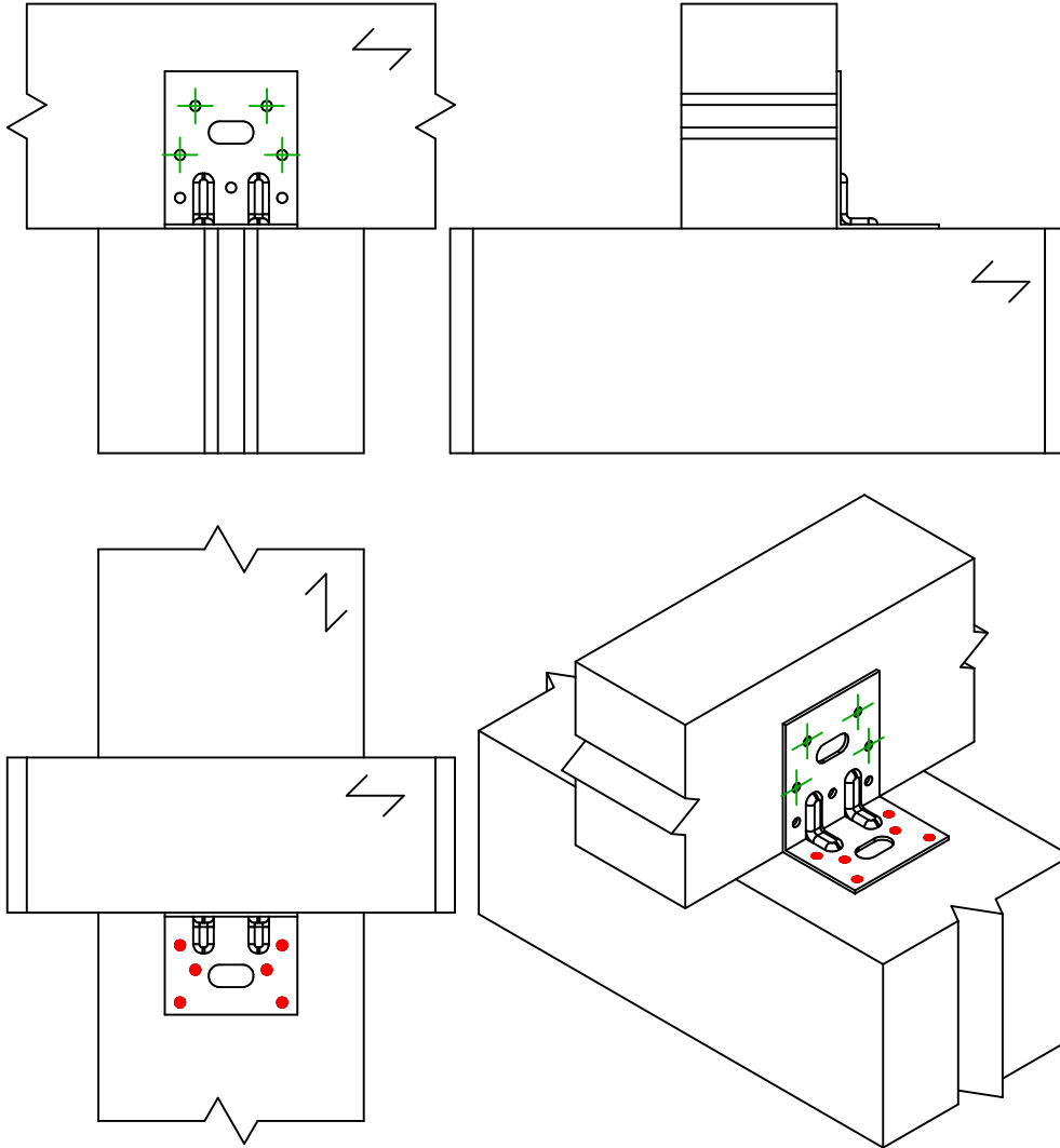
Uitvoering 1 hoekijzer
