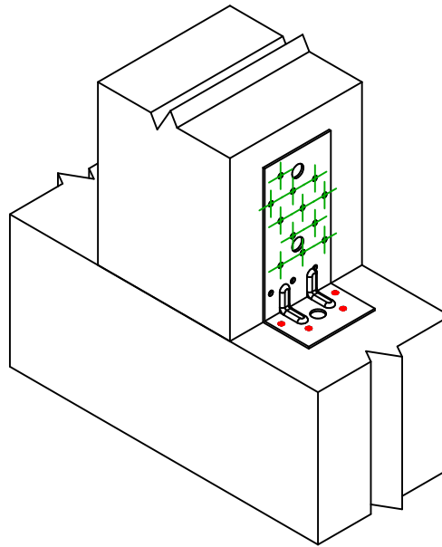
Uitvoering 1 hoekijzer
