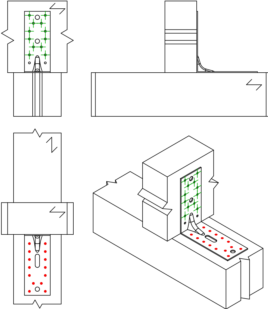
Uitvoering 1 hoekijzer
