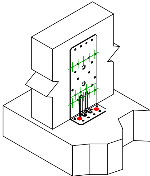
Uitvoering 1 hoekijzer
