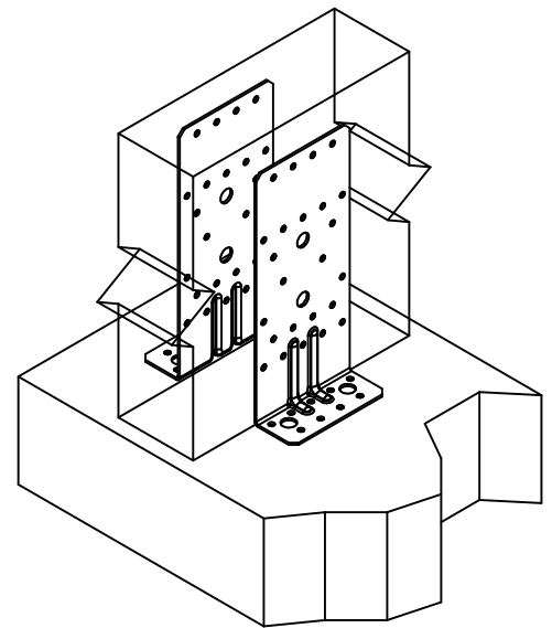
Uitvoering 2 hoekijzers
