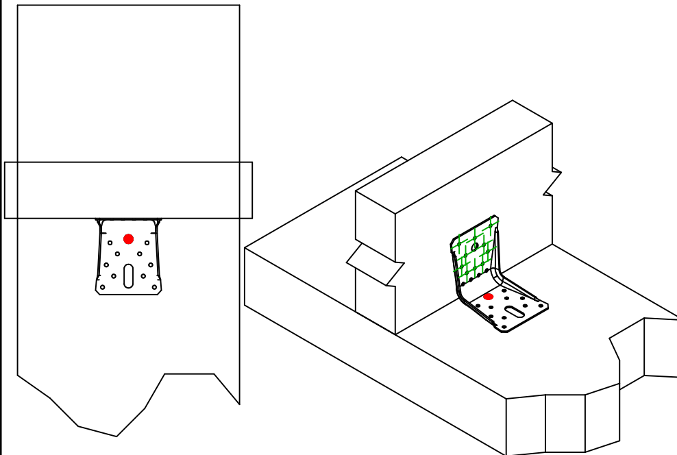
Uitvoering 1 hoekijzer
